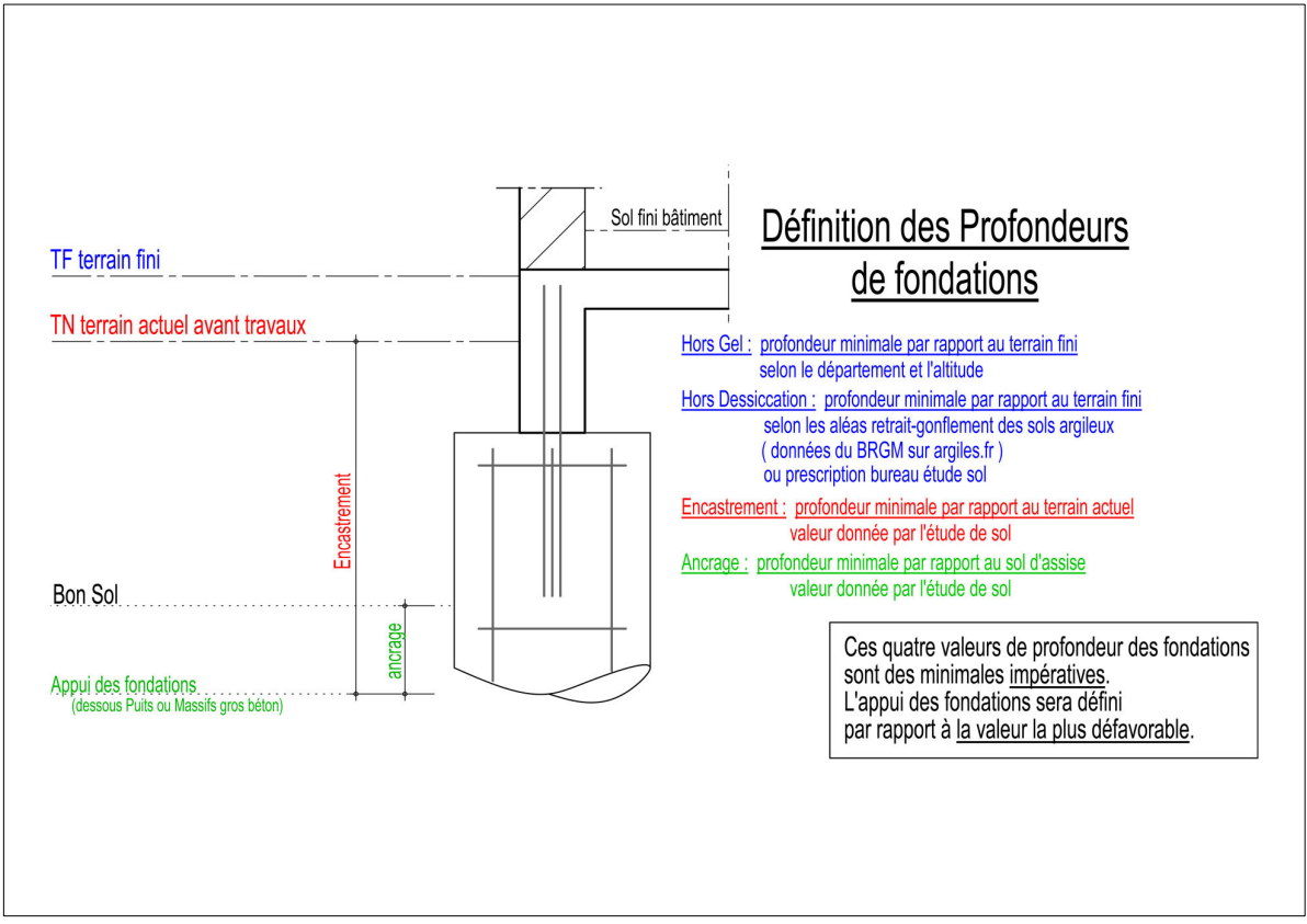
Schéma de principe des fondations profondes
